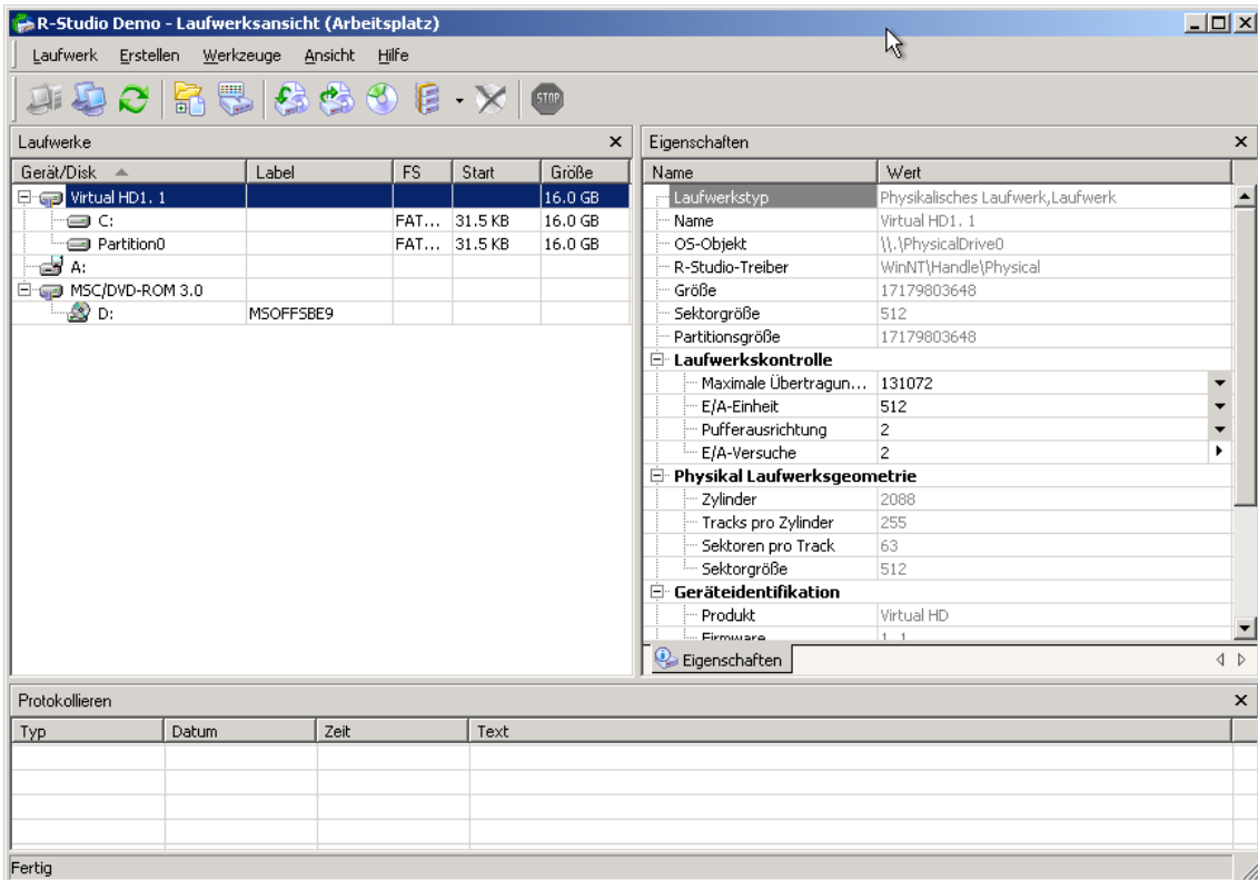
R-Studio 3 Startbildschirm
